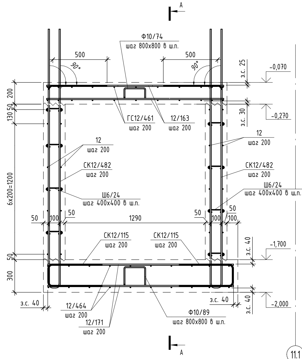
Армирование
