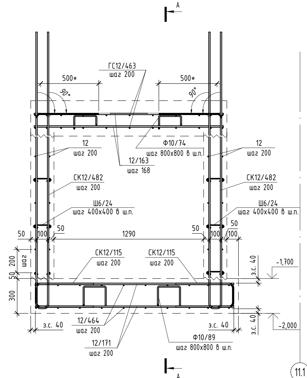
Армирование
