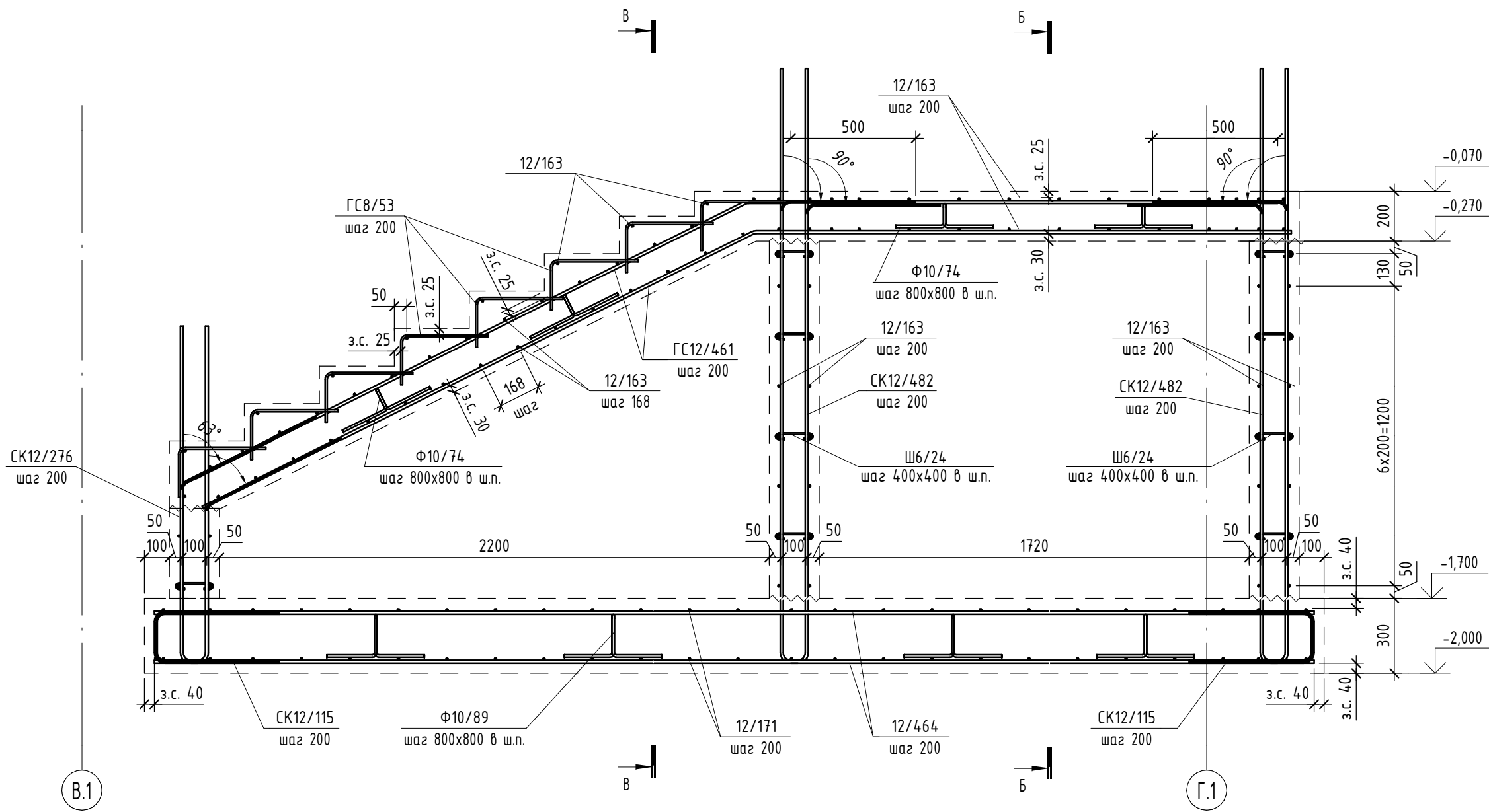
А-А Армирование
